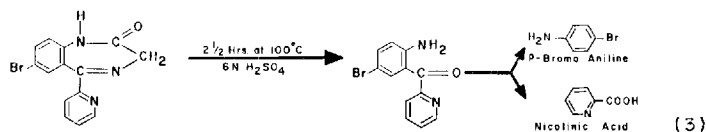
Ro 5-3350
